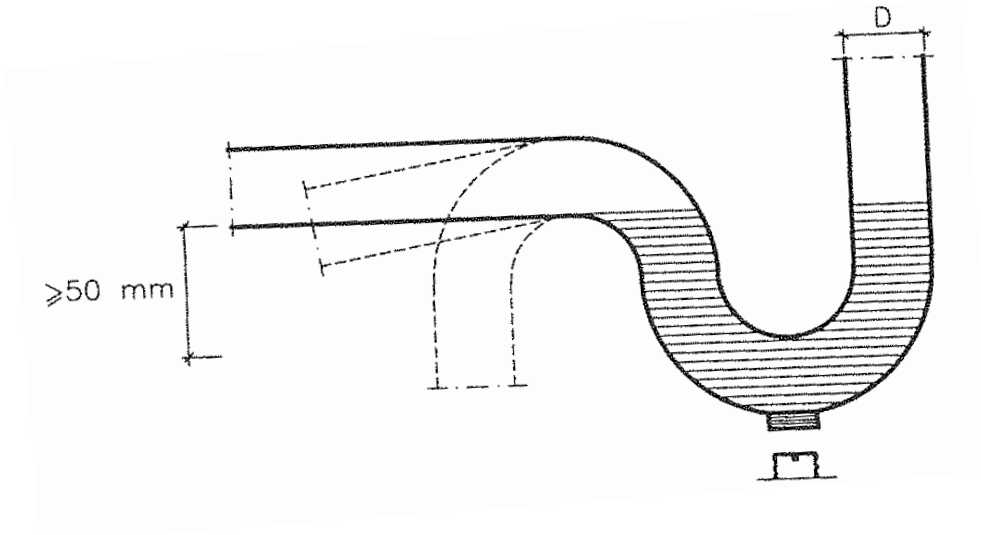
Figura 46. Sifón.
